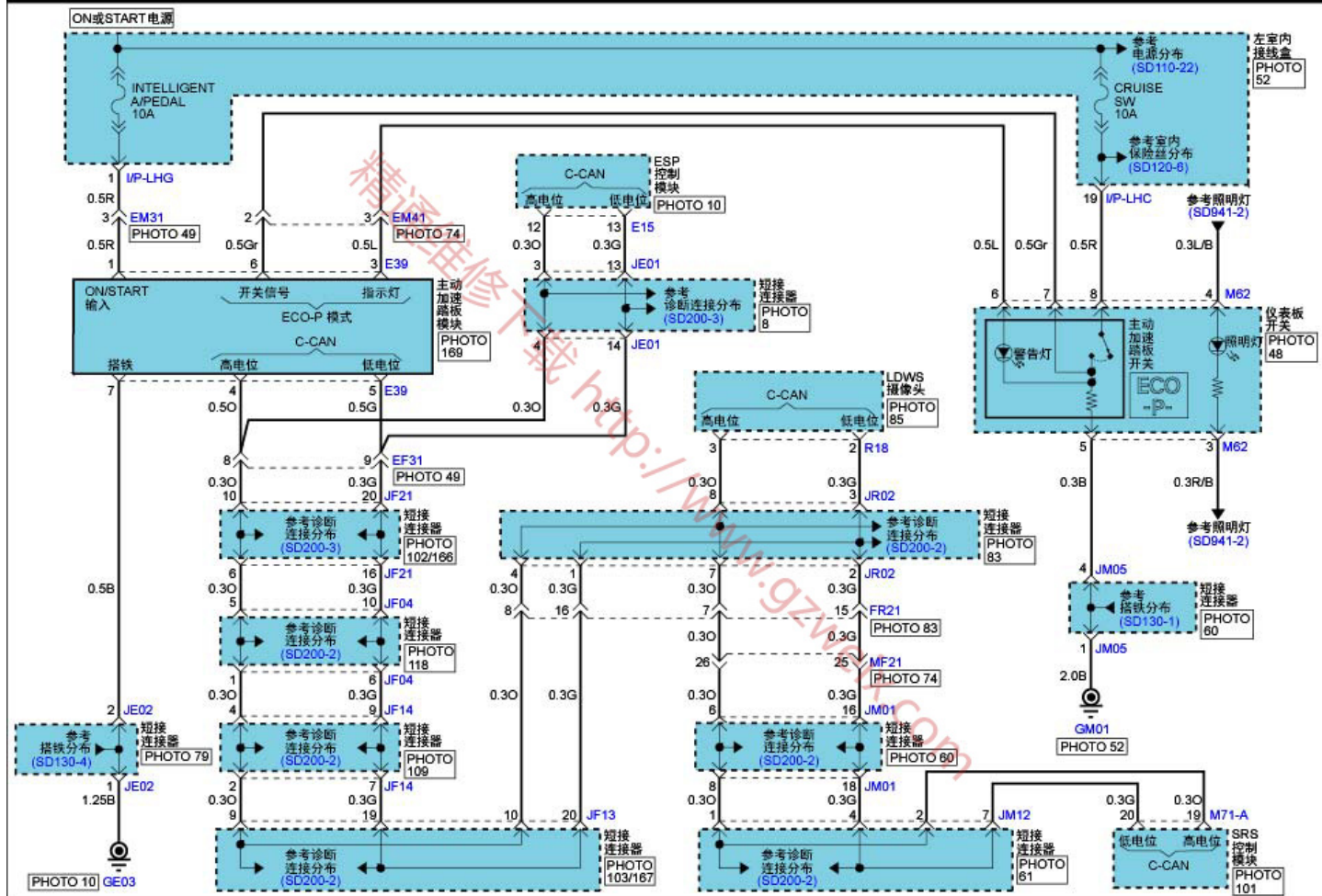
智能加速踏板(IAP)系统(1)
